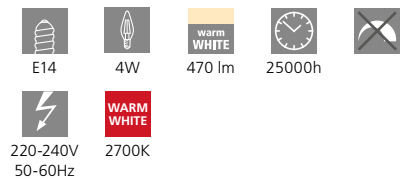
11602 4W E14 CANDLE
