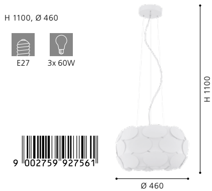
92756 MONTORIO pendant luminaire; steel, white
