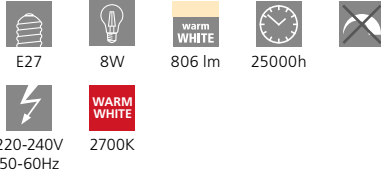
11596 8W E27 GLS
