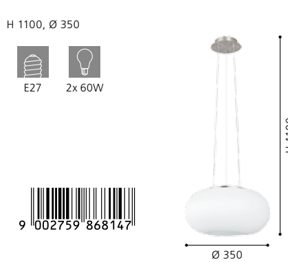
86814 OPTICA pendant luminaire; steel, satin nickel / opal glass
