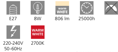
11601 8W E27 G95
