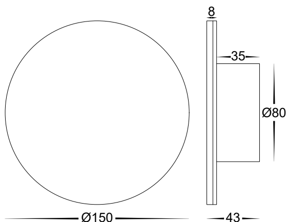
Dimensions
