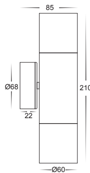
Dimensions
