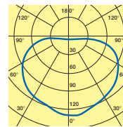
Cod. 3000 piano orizzontale horizontal plane
