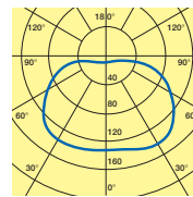
Cod. 3001 piano orizzontale horizontal plane
