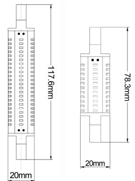
R71A, R72A
