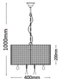
GEM3-R Round Black 3xE14 Iron/PVC shade/ Crystal/Glass D: 400mm H: 1000mm
