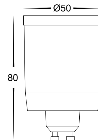
Dimensions
