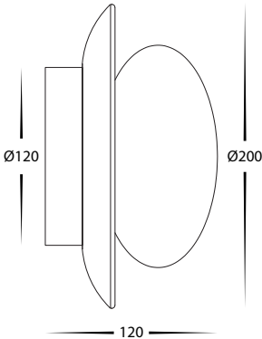
Dimensions
