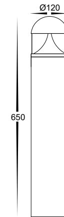
HV1632T Dimensions
